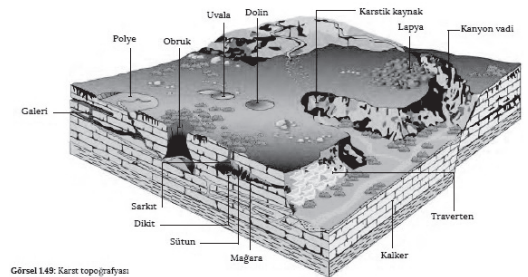
Görsel 148: Karst topografyası
